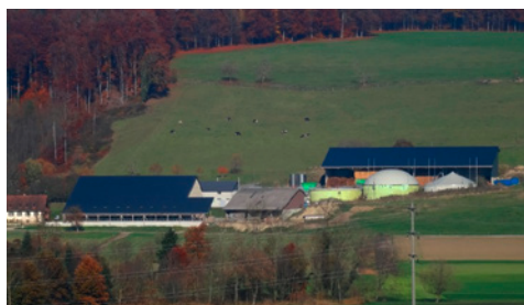
Biogasanlage in Seedorf (Noréaz) mit einer elektrischen Leistung von 295 kW. Quelle: Marcel Gutschner
