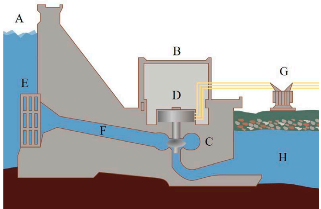
Schema eines Wasserkraftwerks.
