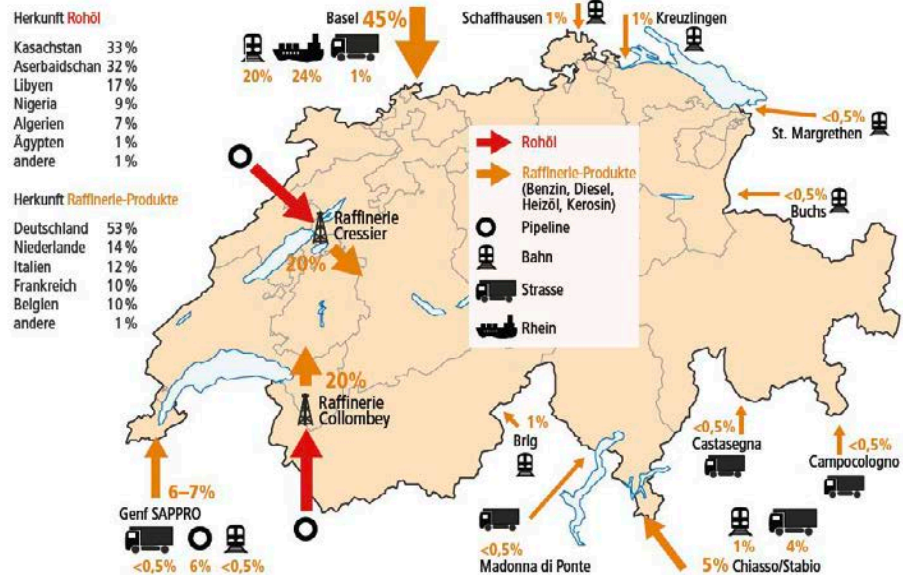
Mineralölimporte 2010. Die Raffinerie in Collombey ist ausser Betrieb. Quelle: BWL
