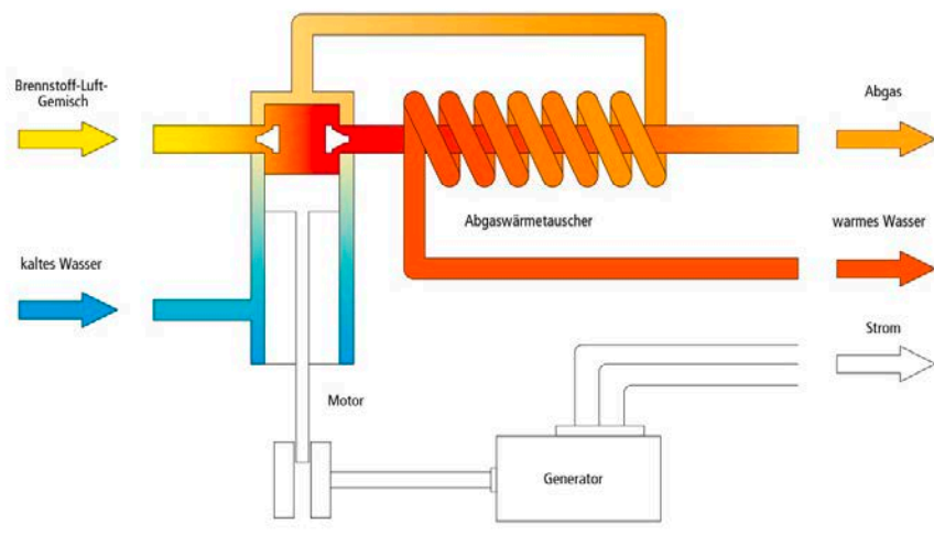
Funktionsweise der Wärme-Kraft-Kopplung. Quelle: VSE
