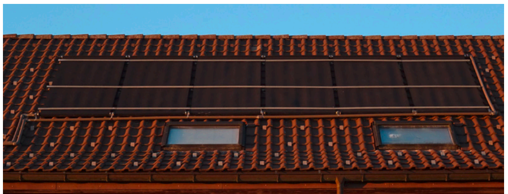
Kollektoren mit Kunststoffabsorber in Alterswil, häufig verwendet zur Wassererwärmung von Schwimmbädern im Freien. Quelle: Marcel Gutschner
