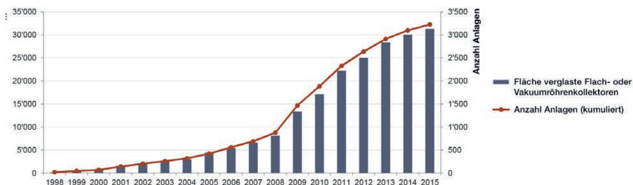
Fläche und Anzahl der im Kanton Freiburg eingebauten thermischen Solaranlagen
