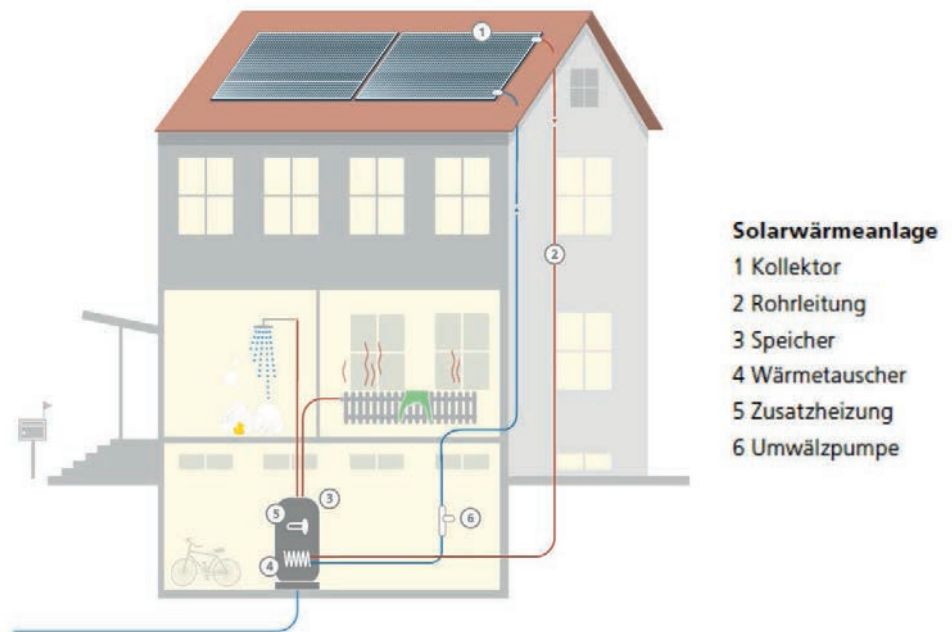
Schema einer thermischen Solaranlage für Warmwasser und Raumwärme. Quelle: Swissolar (2015) [4]
