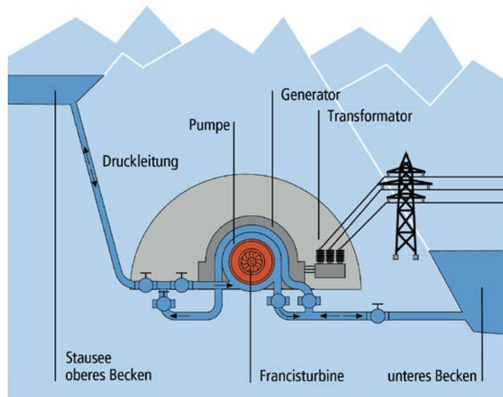
Schema eines Pumpspeicherkraftwerks. Quelle: http://www.fmv.ch/images/pompage-turbinage.jpg
