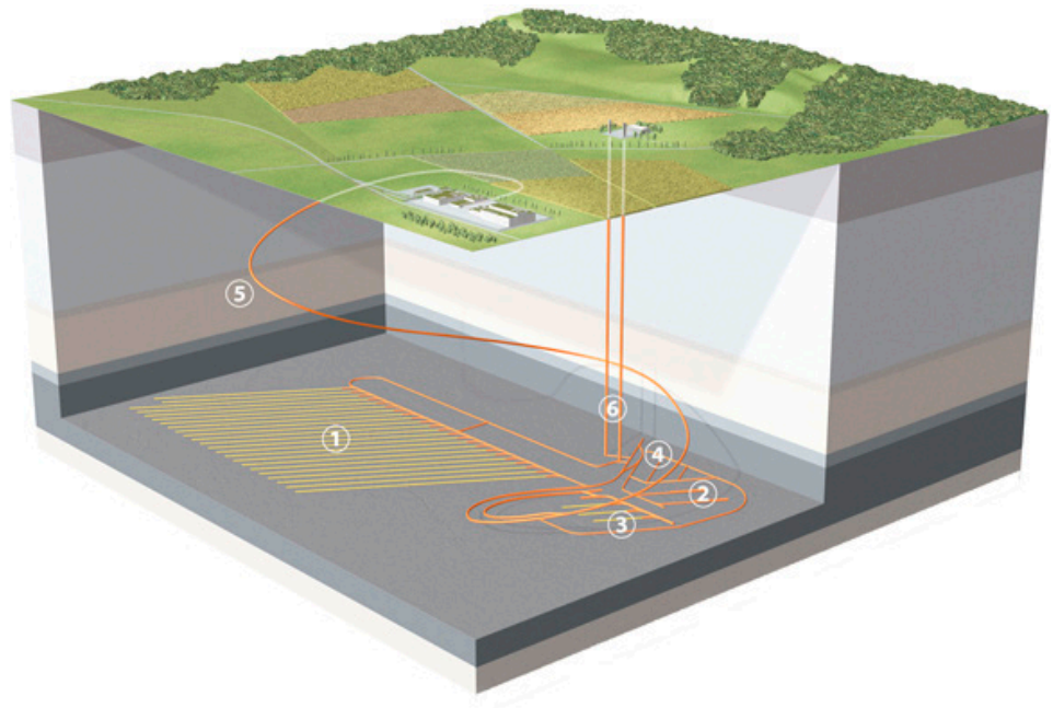
Lager für hochradioaktive Abfälle. Quelle: Nagra
