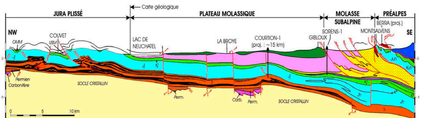
Geologische Situation des Kantons Freiburg (Quelle: Universität Neuenburg – CHYN)
