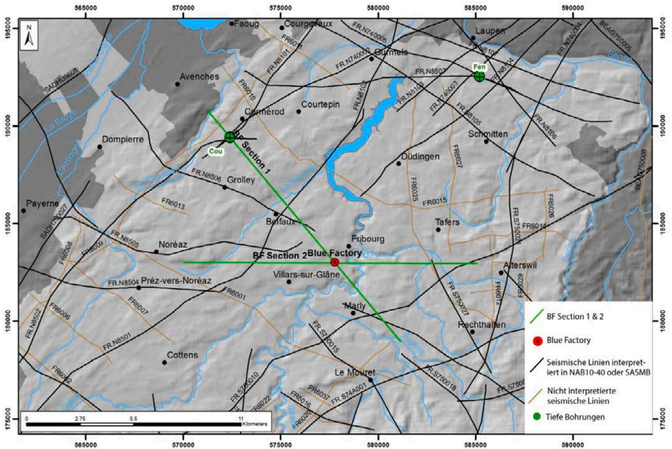
Beispiel von Studienresultaten [11]: Seismische Linien und Einzeichnung der Schnitte, die durch das blueFACTORY-Gelände führen
