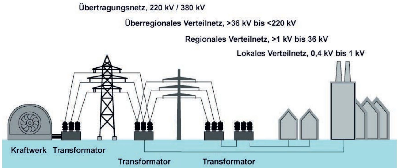
Die verschiedenen Ebenen des Schweizer Stromnetzes. Quelle: VSE (2011)
