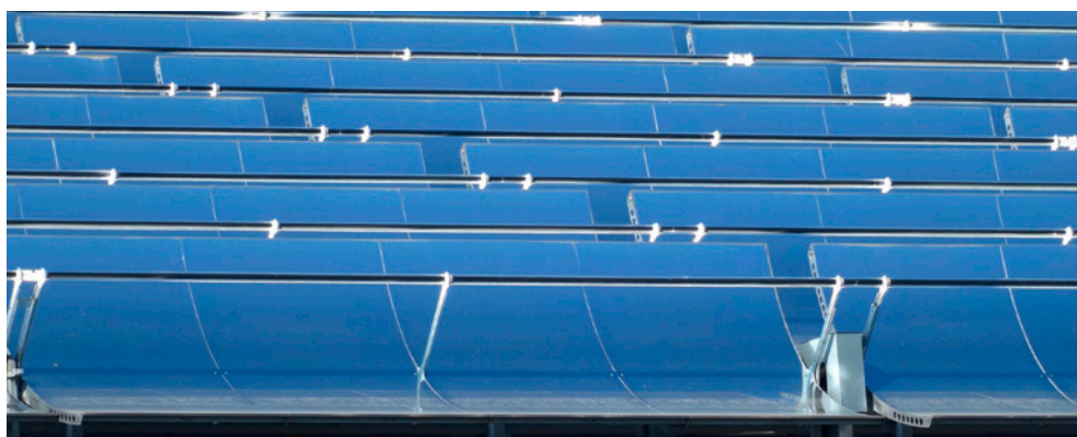
Konzentrierende Kollektoren auf dem Dach eines Milchverarbeitungsunternehmens in Villars-sur-Glâne. Quelle: Marcel Gutschner
