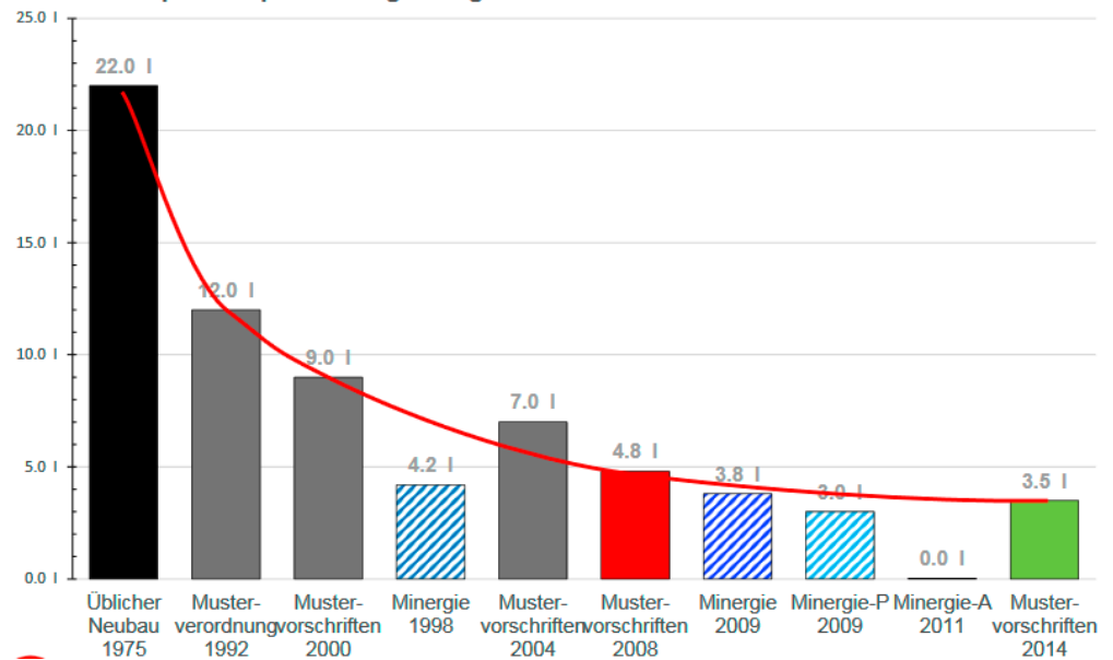
Liter Heizöl-Äquivalent pro m 2 Energiebezugsfläche und Jahr
