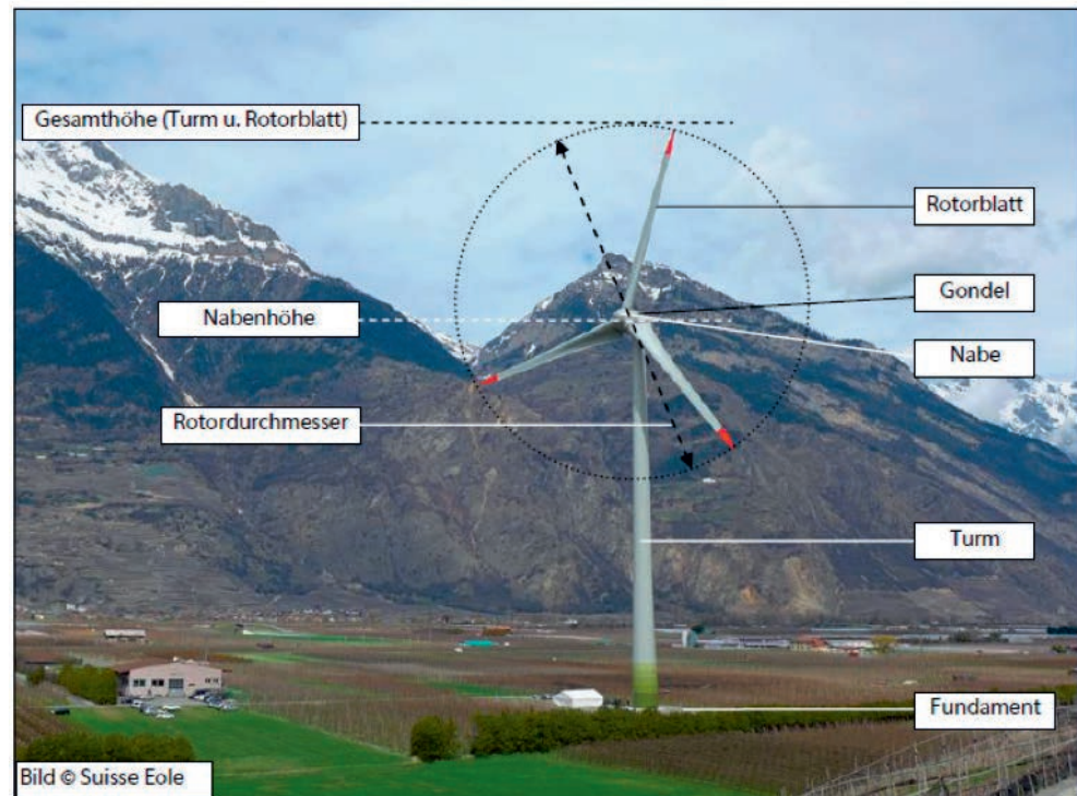
Bestandteile einer Windenergieanlage am Beispiel der Anlage von Charrat (VS).
