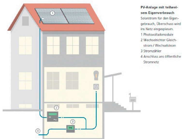
Photovoltaikanlage mit teilweise Eigenverbrauch. Quelle: Swissolar (2015) [4]
