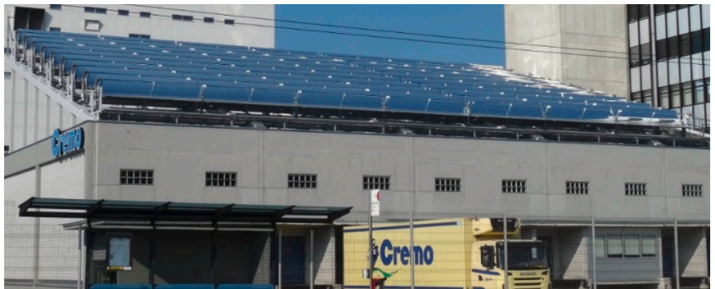
Dieses Milchverarbeitungsunternehmen in Villars-sur-Glâne verfügt über eine Anlage mit einer Kollektorfläche von 580 m 2 (konzentrierende Kollektoren). Die Anlage dient zur Erwärmung des Wassers auf 150 °C für die Sterilisierung von Rahm. Quelle: Marcel Gutschner
