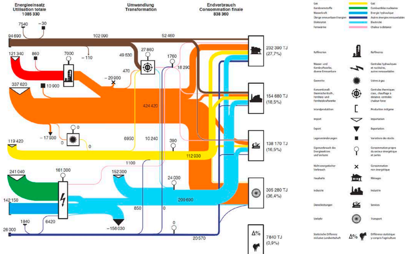
Der Energiefluss in der Energieversorgung der Schweiz. Quelle: BFE (2016) [2]
