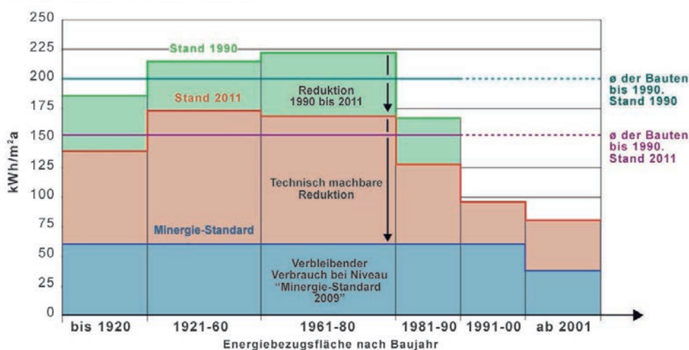
Energieverbrauch von bestehenden Gebäuden nach Baujahren:
