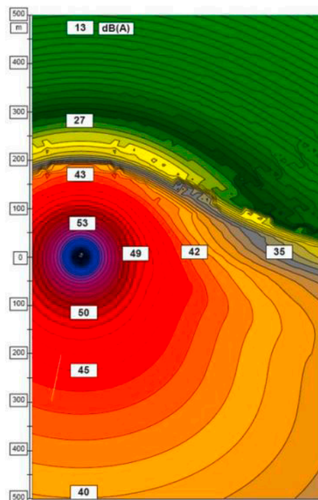
Die Schallausbreitung einer Windenergieanlage hängt stark von der Topografie und der Windrichtung ab: Der blau-schwarze Punkt ist der Standort der Anlage. Die Gebiete mit ähnlichem Schallpegel sind mit gleicher Farbe gekennzeichnet. Quelle: Suisse Eole
