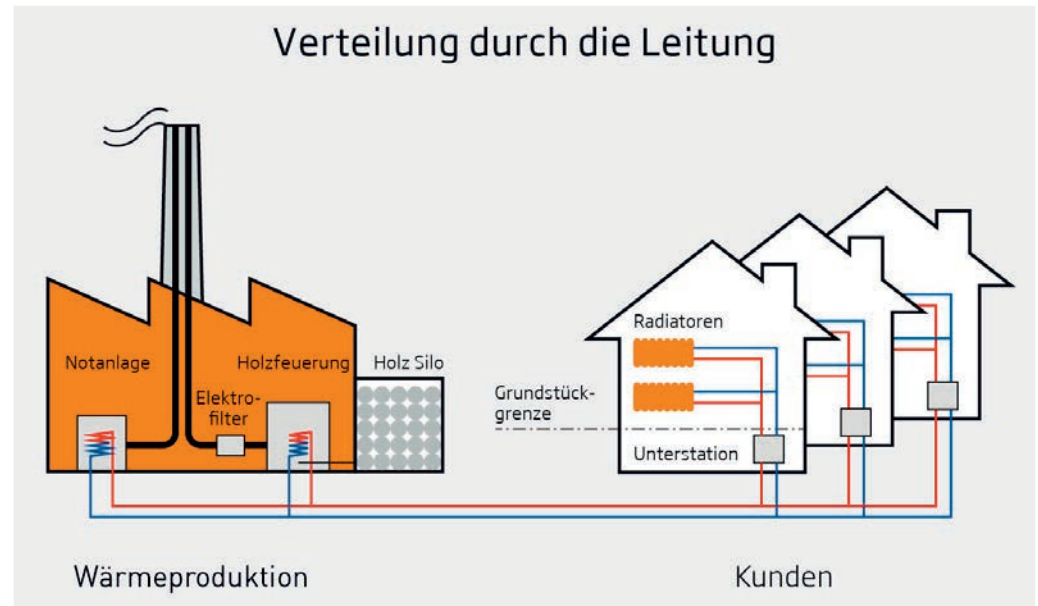
Schema einer Fernheizung. Quelle: Groupe E
