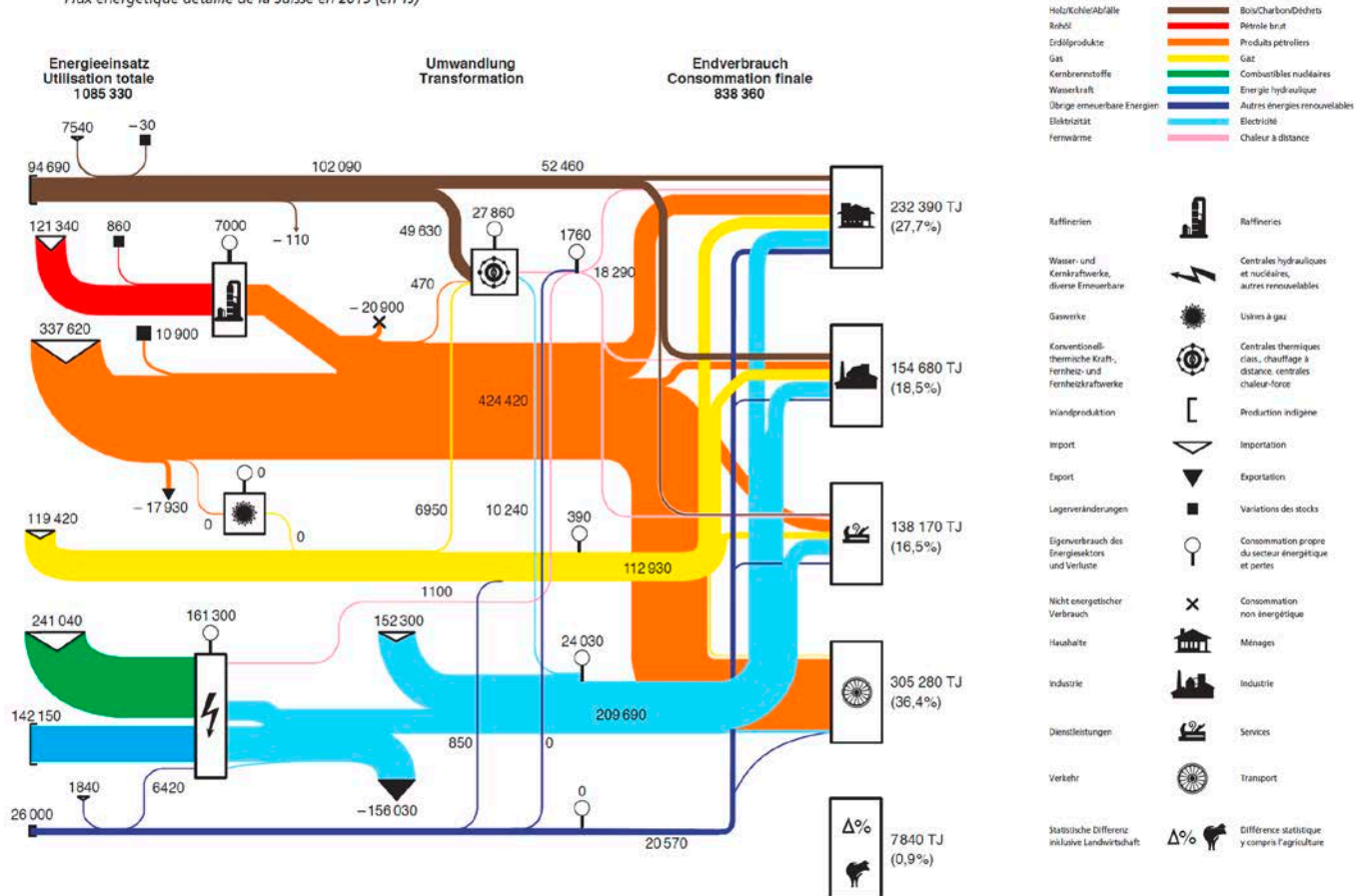
Flux énergétique détaillé de la Suisse en 2015 (en TJ)
