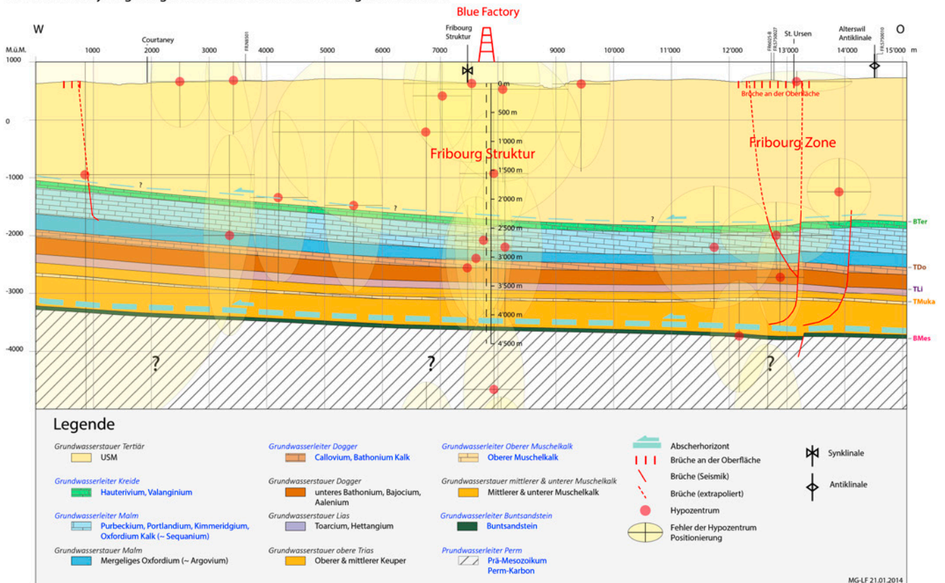
Beispiel von Studienresultaten [11]: Geologischer Schnitt am voraussichtlichen Bohrstandort auf dem blueFACTORY-Gelände
