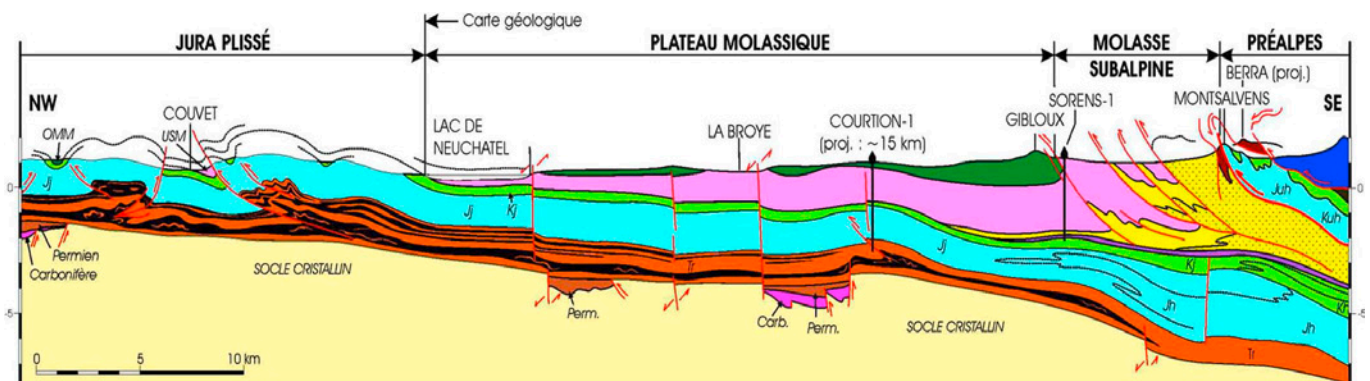
Geologische Situation des Kantons Freiburg (Quelle: Universität Neuenburg – CHYN)
